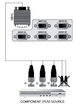
DB15 or 3xBNC
